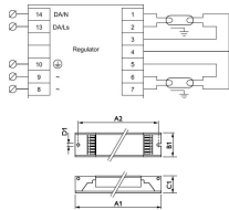
Technische Daten Philips HF-Ri TD 2 28-54 TL5 E+ 195-240V
